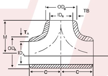
TEES
